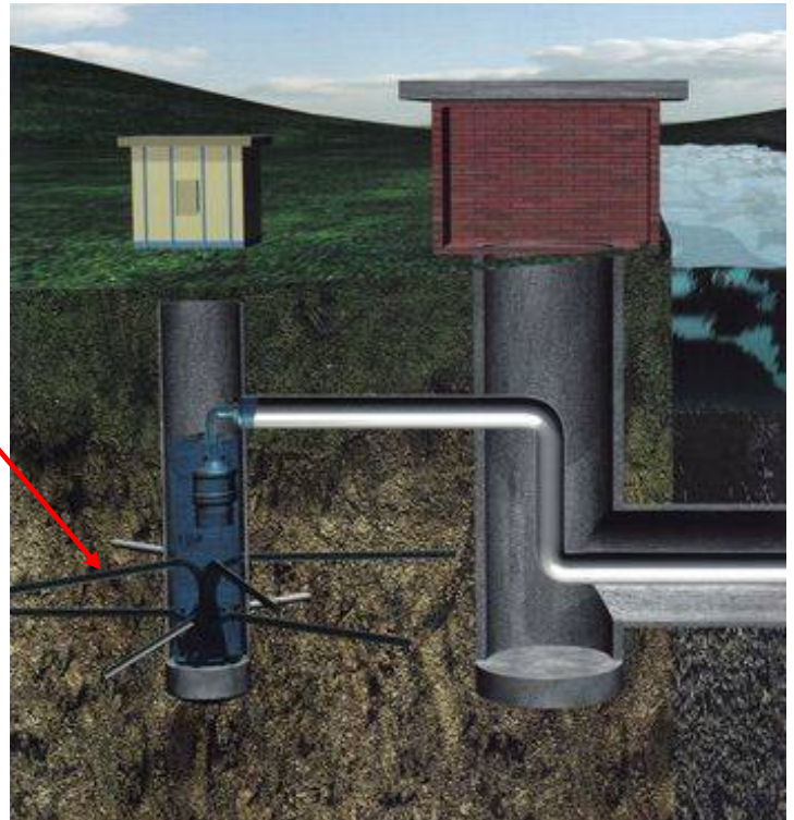
Egy csáposkút rajza
